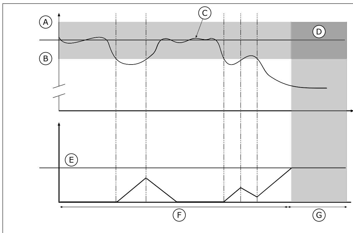
Σχ. 83: Η λειτουργία επίβλεψης ανάδρασης
