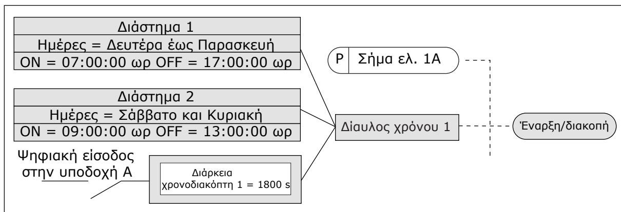
Σχ. 78: Το κανάλι χρόνου 1 χρησιμοποιείται ως το σημείο ελέγχου για την εντολή εκκίνησης, αντί για μια ψηφιακή είσοδο
