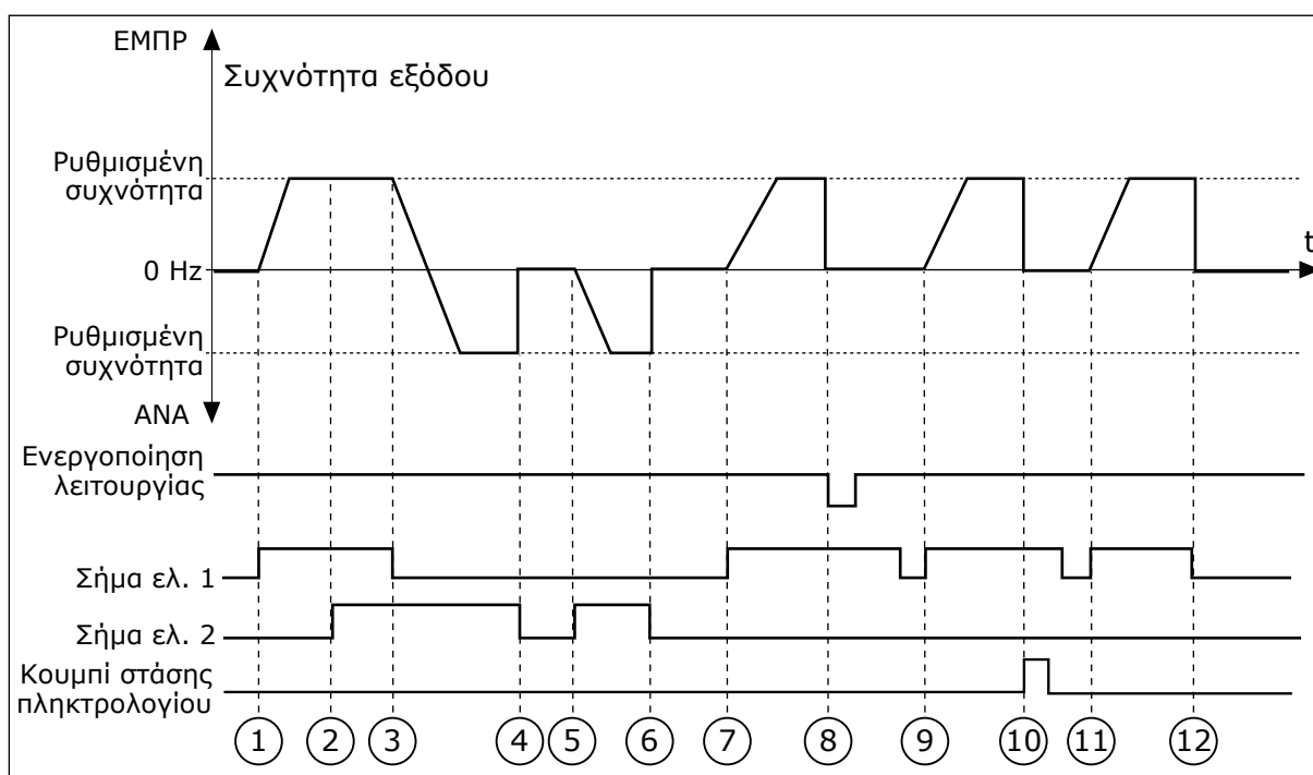
Σχ. 44: Λογική έναρξης/στάσης I / 0 A = 2
