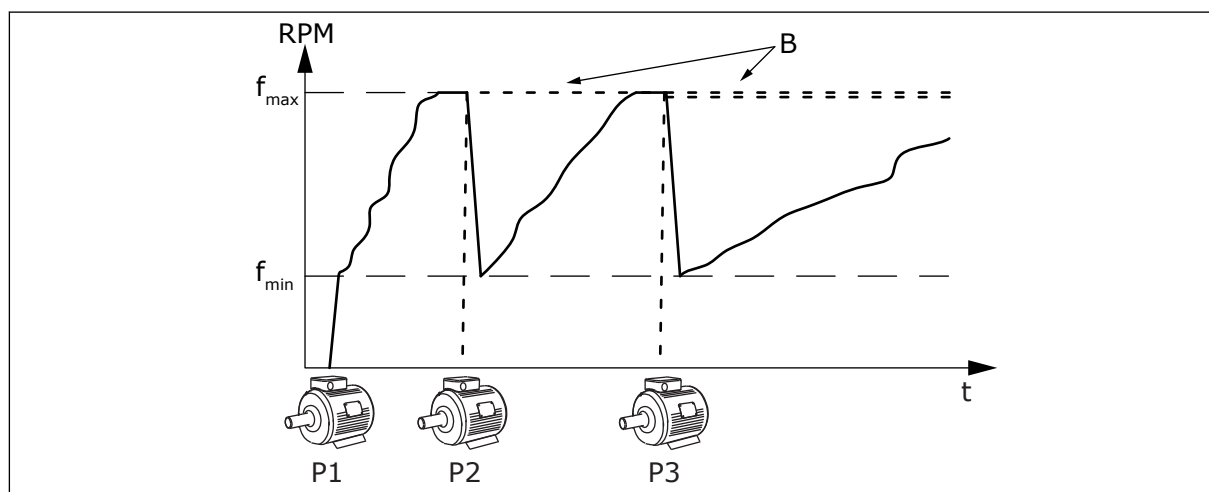
Σχ. 91: Έλεγχος σε λειτουργία ενός ρυθμιστή στροφών
