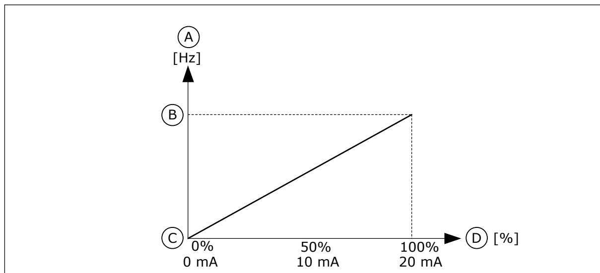
Σχ. 60: Αναστροφή σήματος A/I1, επιλογή 0
