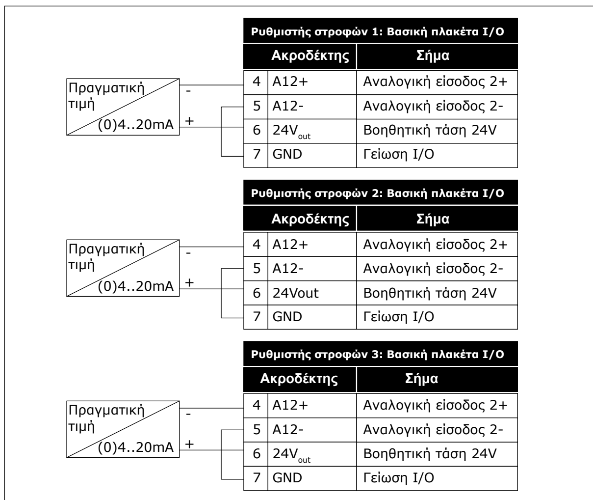
Σχ. 94: Συνδεσμολογία των αισθητήρων ανάδρασης για κάθε ρυθμιστή στροφών
