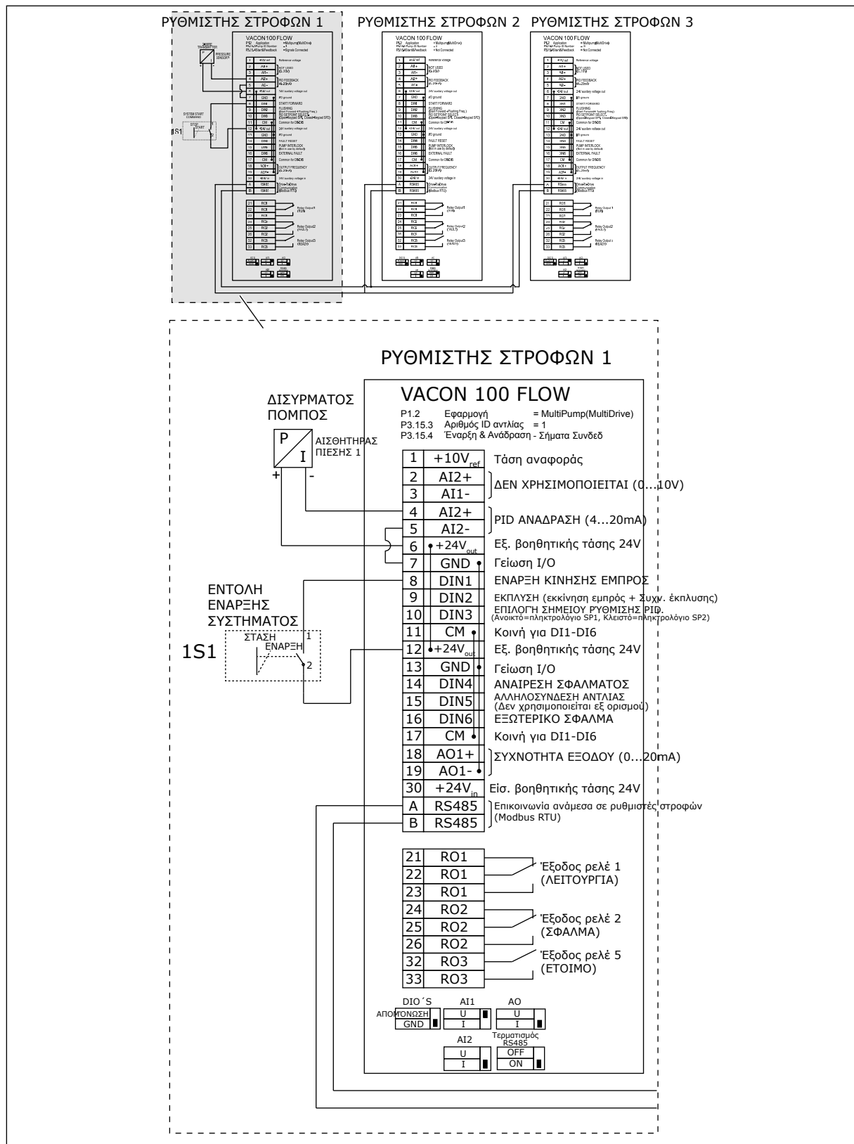
Σχ. 30: Διάγραμμα συνδεσμολογίας του συστήματος πολλαπλών αντλιών (πολλαπλοί ρυθμιστές στρωφών), παράδειγμα 5A
