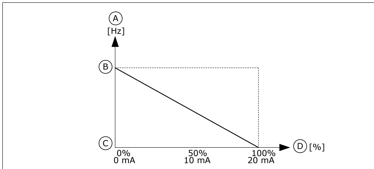
Σχ. 61: Αναστροφή σήματος A/1, επιλογή 1
